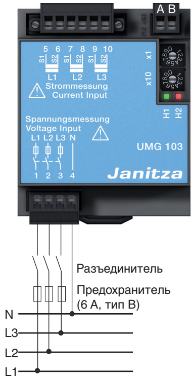
Рис. Пример подключения: измерение напряжения через разъединитель и предохранители.
